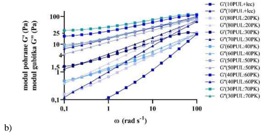
Slika 48. Krivulja ovisnosti: a) modula pohrane ( G' ) i gubitka ( G'' ) o ( \gamma ) smičnoj deformaciji, b) modula pohrane ( G' ) i gubitka ( G'' ) o kutnoj frekvenciji ( \omega ) za otopine na bazi pululana i proteina konoplje.
