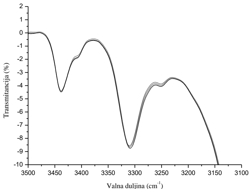
Slika 19. Temperaturno-ovisni IR-spektri spoja 7 u području NH skupina ( \text{CH}_2\text{Cl}_2 , 25-45 °C).
