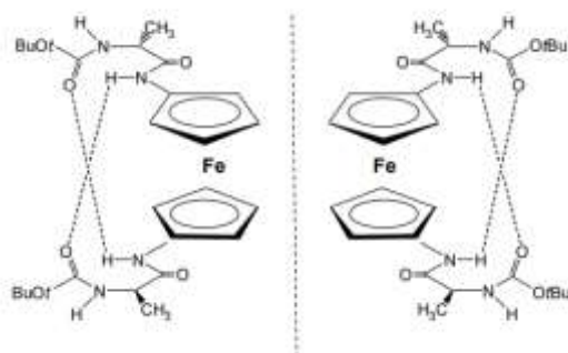
Slika 13. Shematski prikaz IHB dipeptida \text{Fn}-(\text{NH-Ala-Boc})_2 ( VII , lijevo) i \text{Fn}-(\text{NH-D-Ala-Boc})_2 ( VIII , desno)
