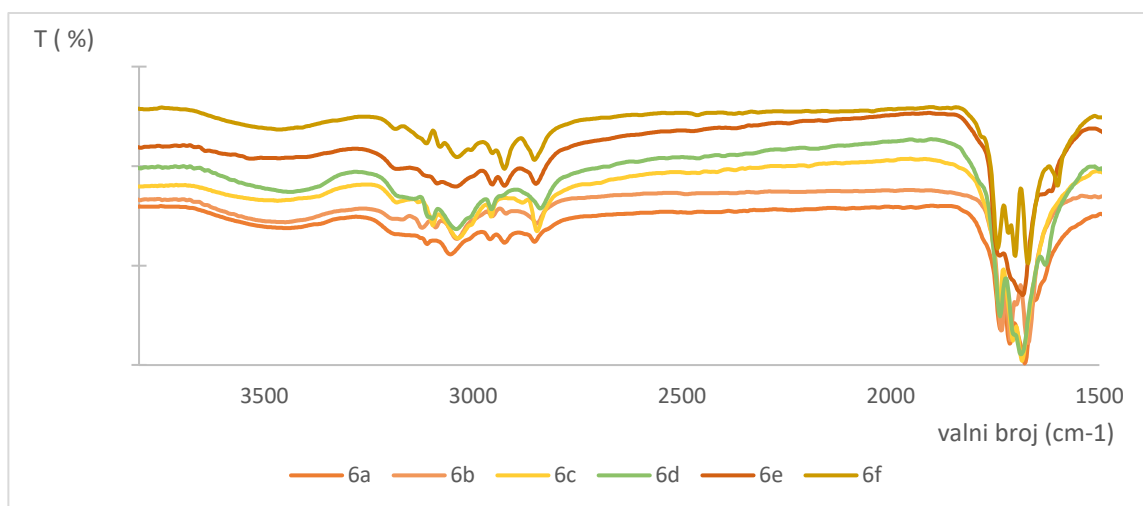
Slika 23. IR spektar spojeva 6a-f
