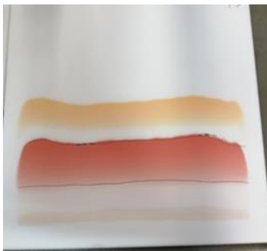
Slika 20. Preparativna tankoslojna kromatografija
