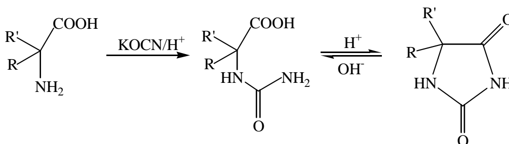
Shema 1. Readova sinteza hidantoina iz \alpha -aminokiselina
