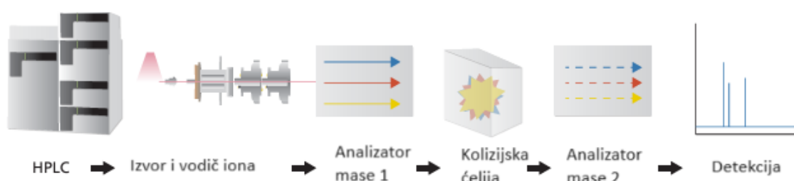
Slika 8. Shematski prikaz tandemske spektrometrije masa LC-MS/MS (prema Ichiro, 2019)
