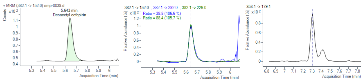
Slika 15. Kromatogram cefaleksina, cefazolina, cefoperazona, cefalonija, cefacetрила, cefkvinoma, ceftiofura, cefapirina i desacetil-cefapirina u uzorku uz-jaja-2 obogaćen na razini od 5 µg/kg - nastavak
