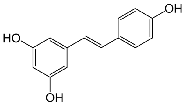
Slika 3. Struktura resveratrola (Anonimus 3)
