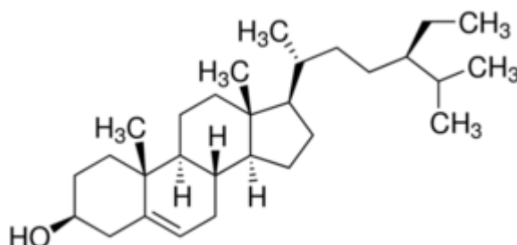
Slika 3. Struktura \beta -sitosterola (Anonymous 3, 2016)
